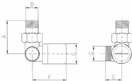
Valvola ad angolo termostattabile versione destra. Right angle radiator valve with thermostatic option.
